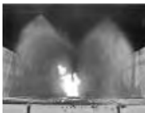
自動車製造ライン 実規模消火実験
