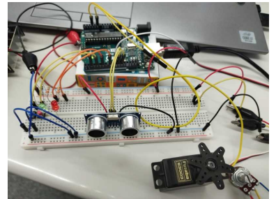
マイコンと周辺回路
