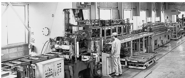
フォーミングライン
