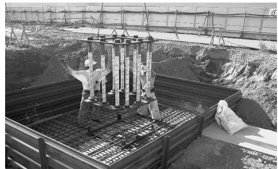
アンカーフレームとセット工事
